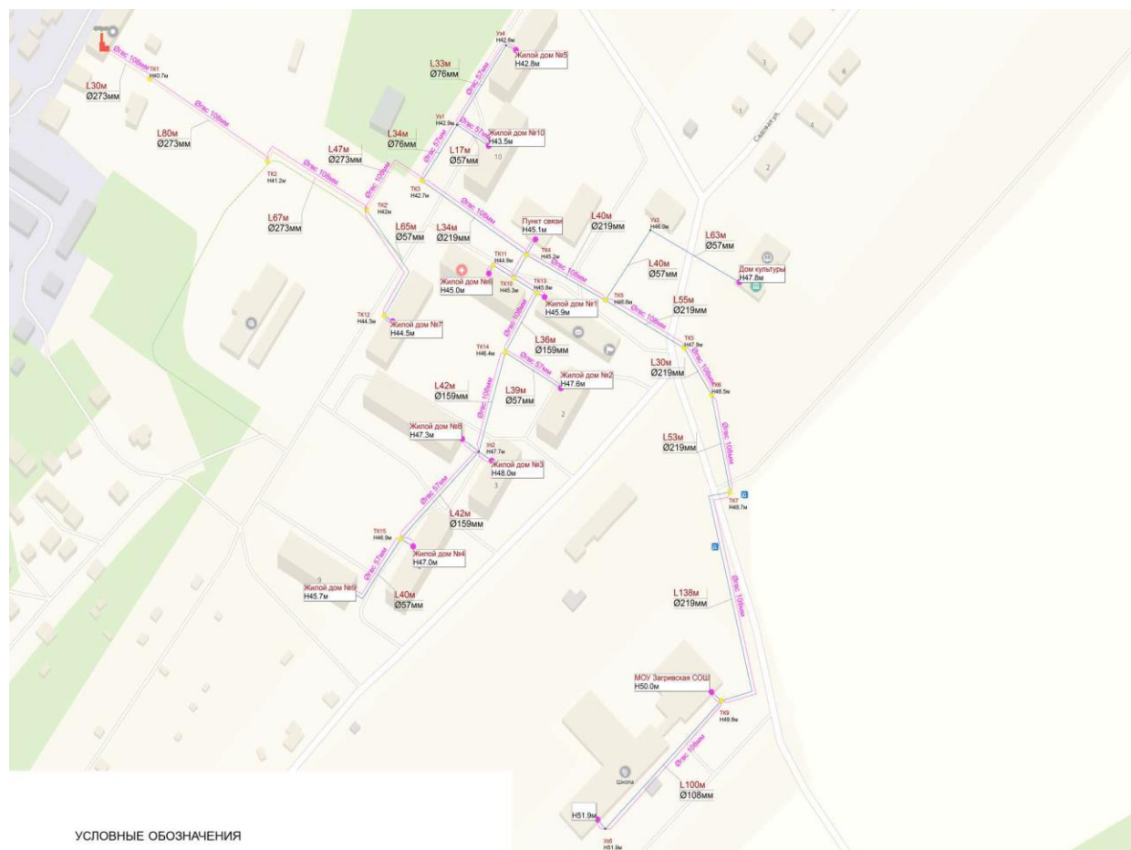
Рисунок 1.3.2.1 - Схема прокладки тепловых сетей от котельной №9
